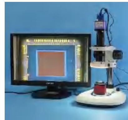
CCD tester
