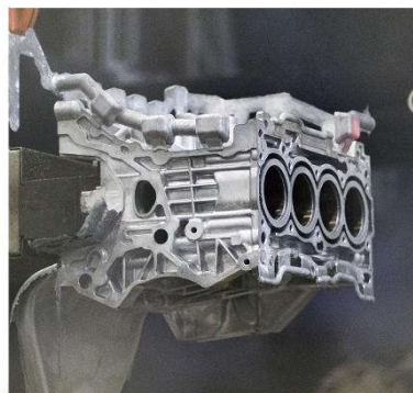
Die casting
